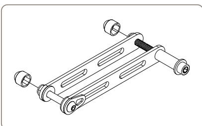
7. 11441 716 Rahmen-/Faltverbinder, rechts
