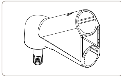
20. 11441 255 Vorderradaufhängung, rechts und links
