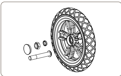
11. 11441 251 Hinterrad mit Lager und Schrauben
