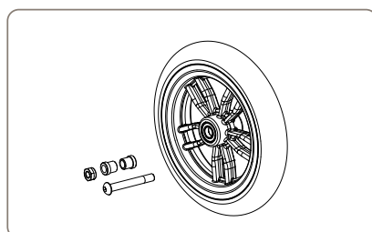
13. 11441 704 Vorderrad mit Lager und Schrauben
