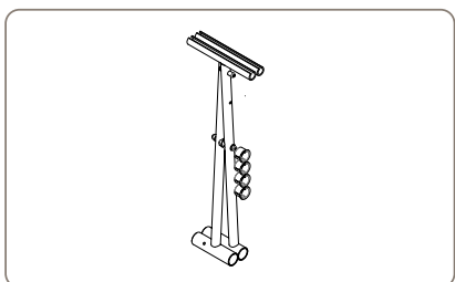
14. 11441 714 Kreuzstrebe, champagner
